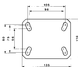
Ø 125/50-150/50
