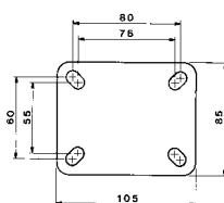
Ø 100-125
