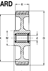
CUSCINETTO A RULLINI STANDARD O INOX - STANDARD OR STAINLESS STEEL ROLLER BEARING - STANDARD ODER ROSTFREIES ROLLENLAGER - ROULEMENT À ROULEAUX STANDARD OU INOX - COJINETE A RODILLOS STANDARD O INOX
